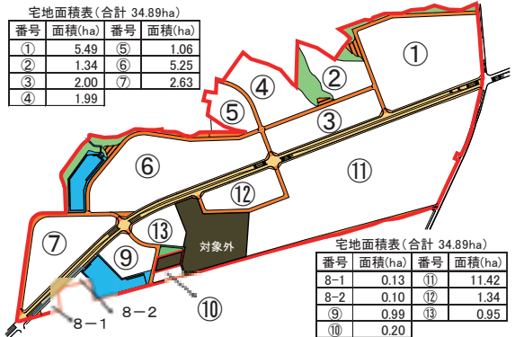
区画予定図
